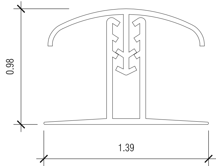
1 SIDE VIEW scale: 2:1
