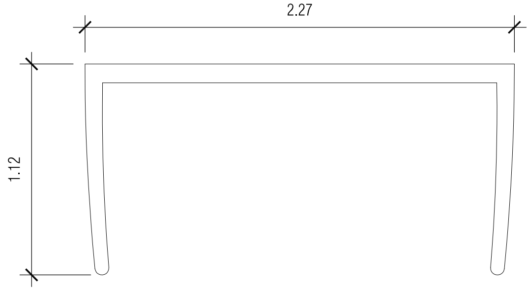
1 SIDE VIEW scale: 2:1
