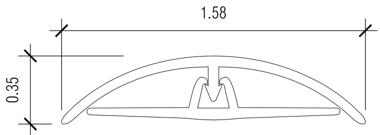
1 SIDE VIEW scale: 2:1
