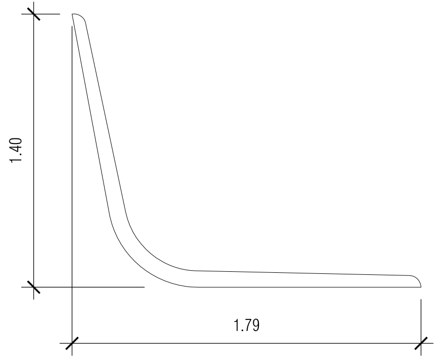
1 SIDE VIEW scale: 2:1
